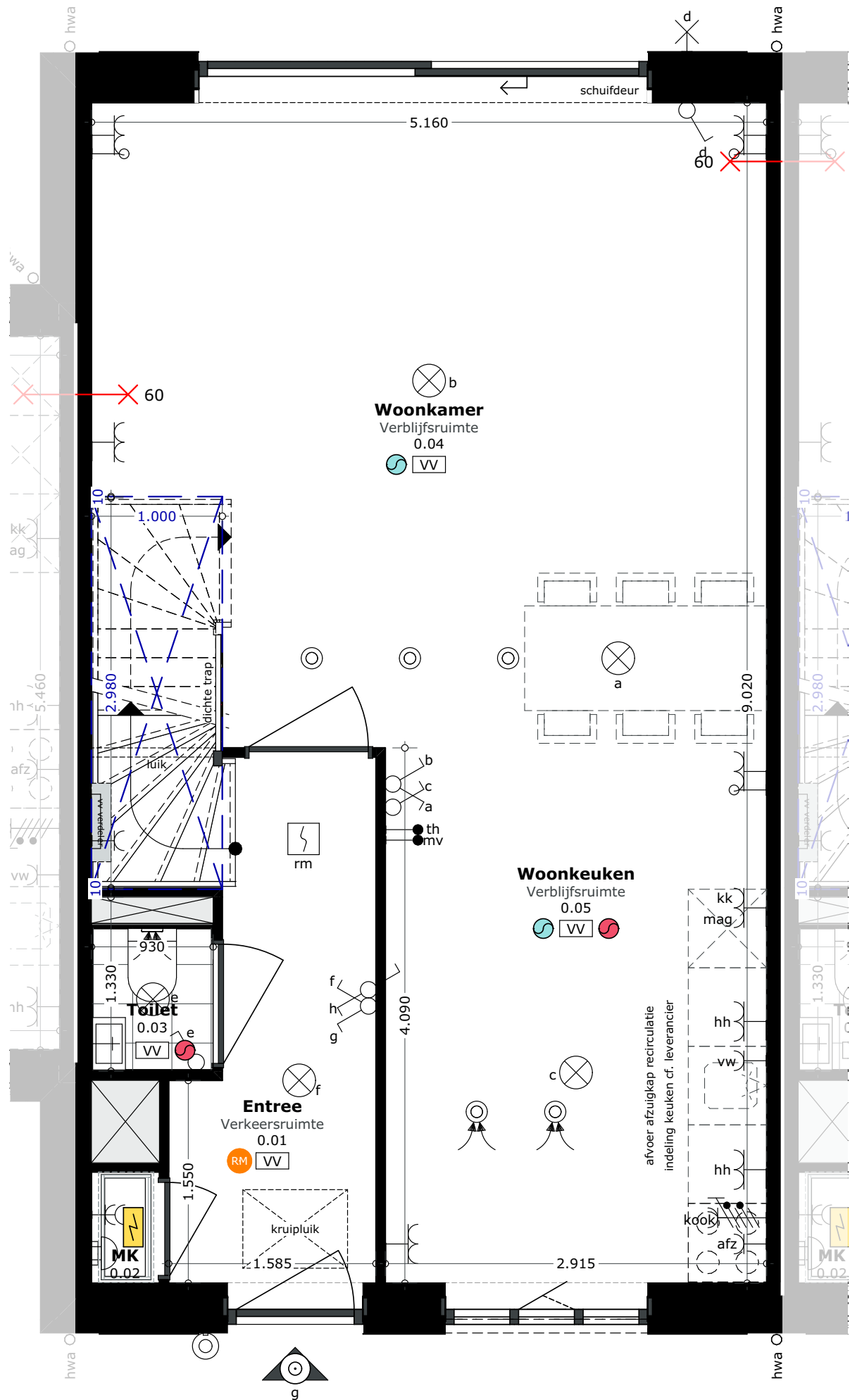
Begane grond
