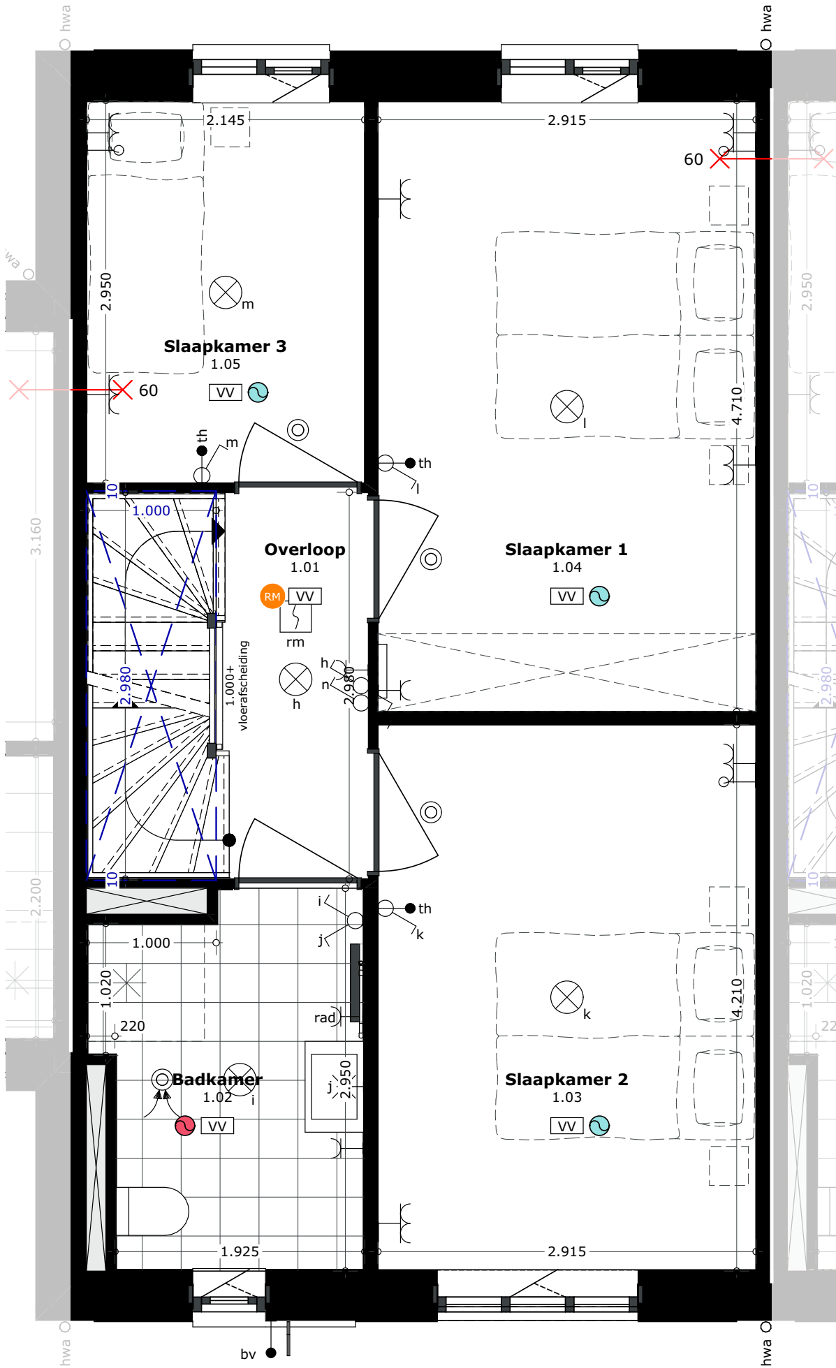
1e Verdieping
