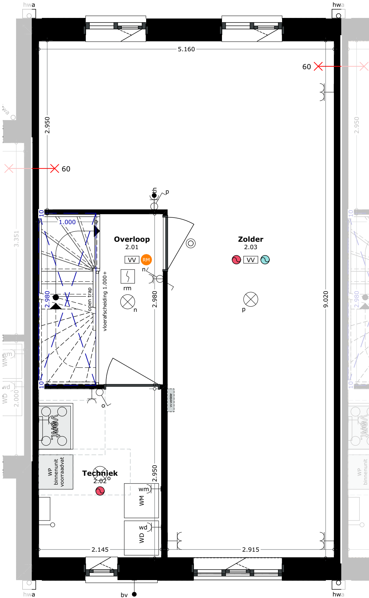
2e Verdieping
