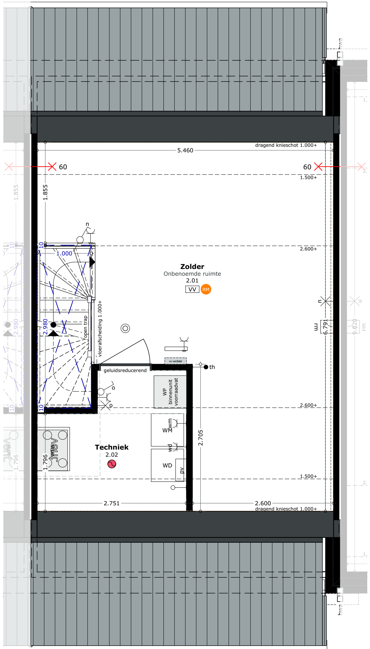
Tweede verdieping
