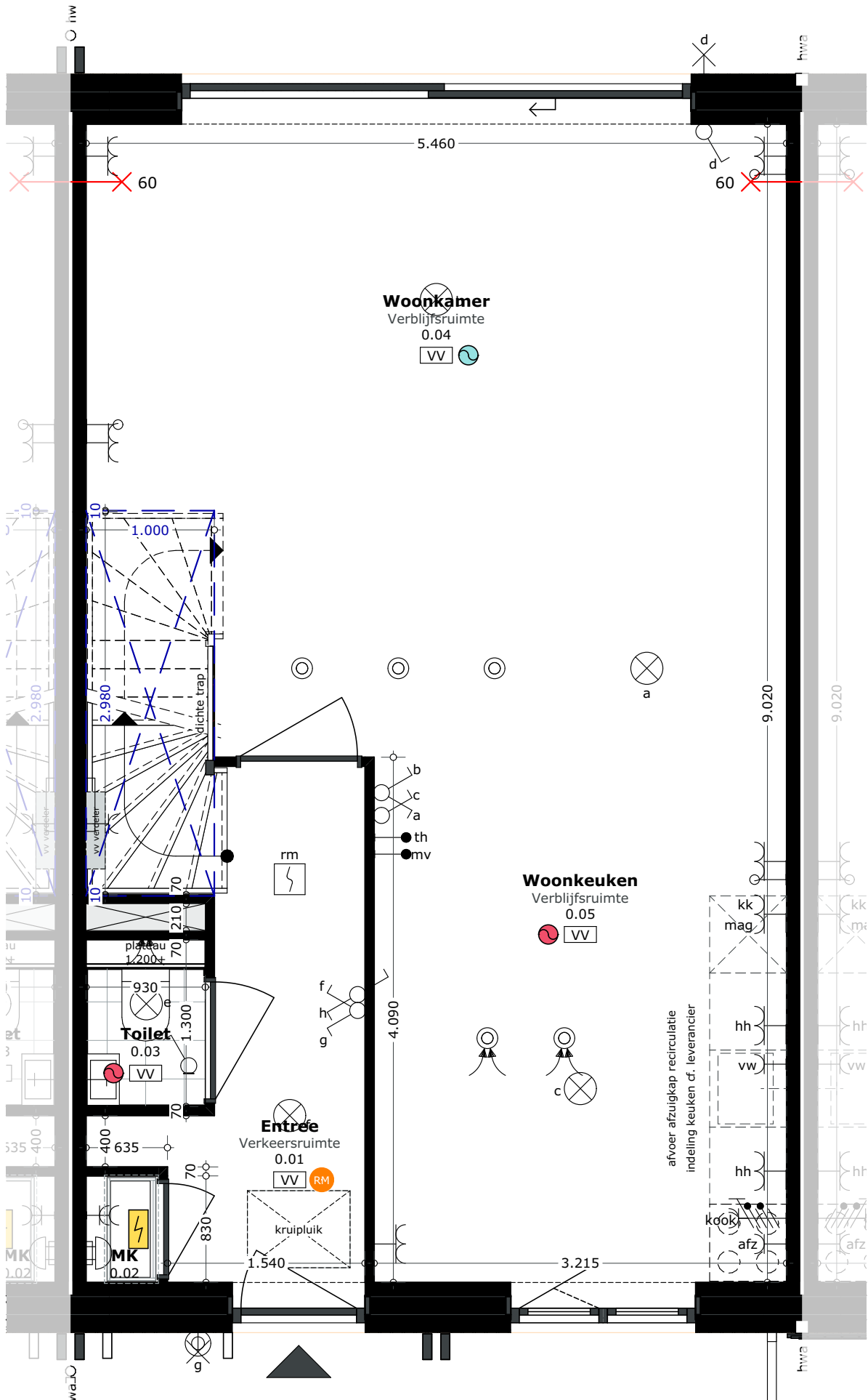
Begane grond
